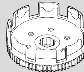
CAMPANA DE EMBRAGUE
