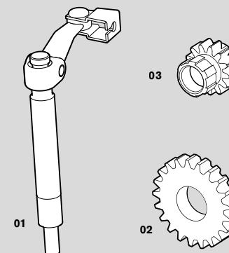
VARILLA DE EMPUJE
